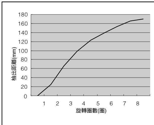
E3X-ZA11
